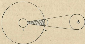
ECLIPSE TOTAL DE SOL. — La luna (L) se interpone entre el Sol (S) y la Tierra (T) impidiendo completamente que los habitantes de una parte de la Tierra puedan ver el Sol.
